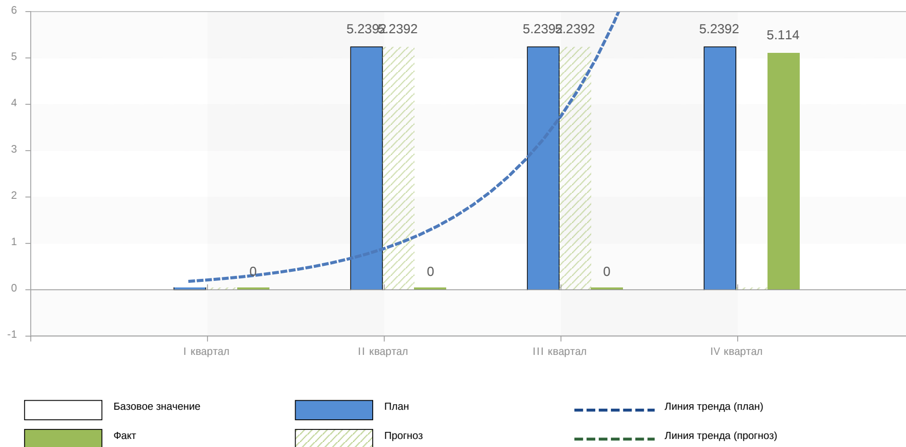
Рис. 12. Ущерб от лесных пожаров по годам
