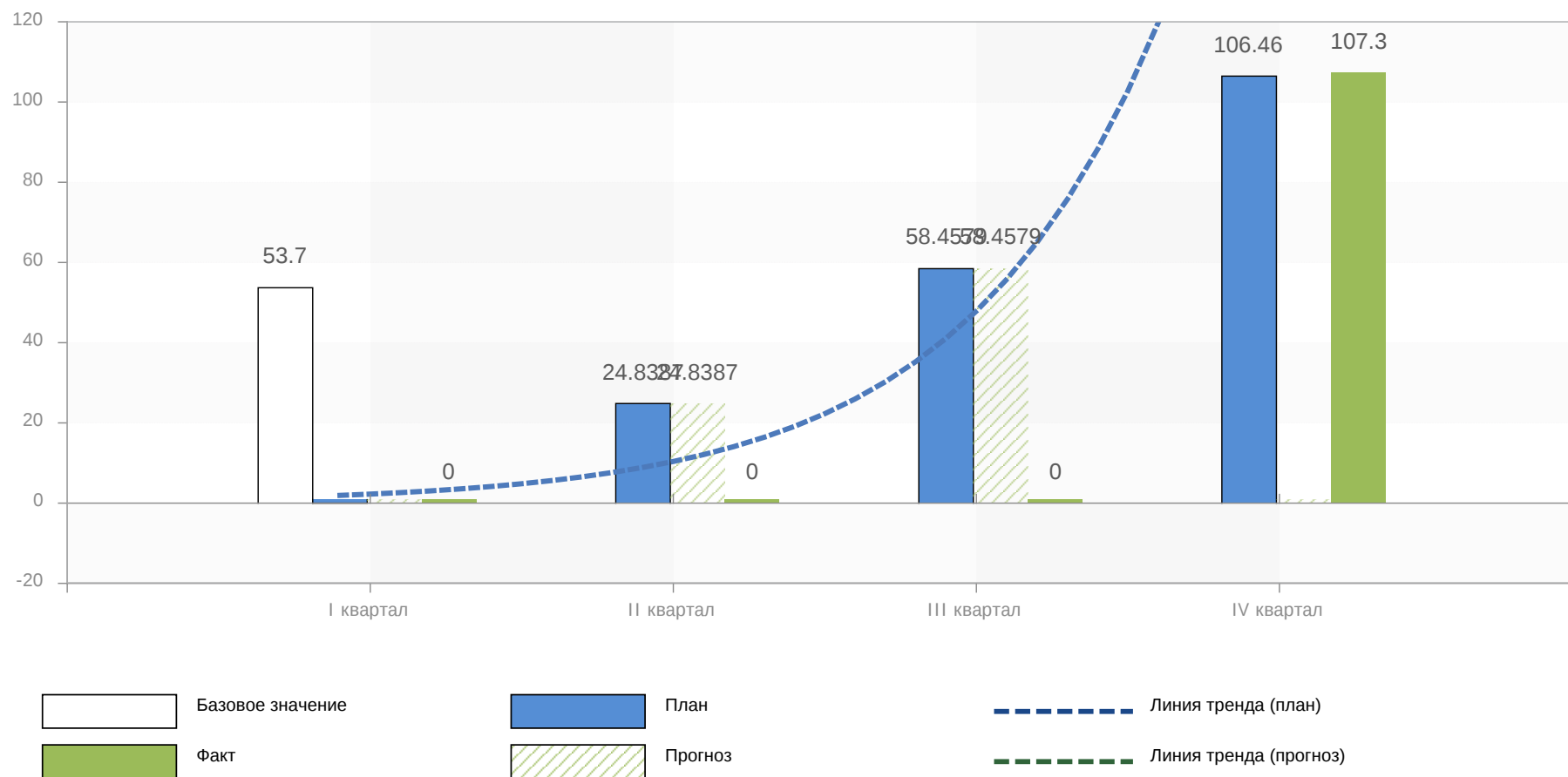
Рис. 6. Отношение площади лесовосстановления и лесоразведения к площади вырубленных и погибших лесных насаждений
