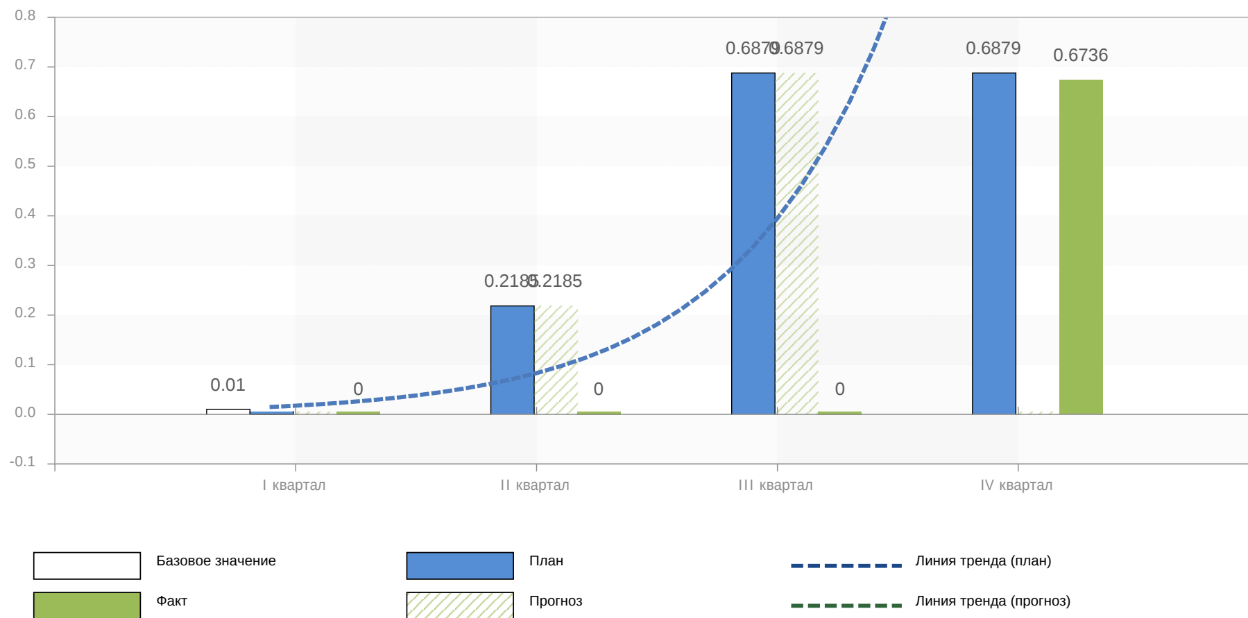
Рис. 10. Площадь погибших лесных насаждений
