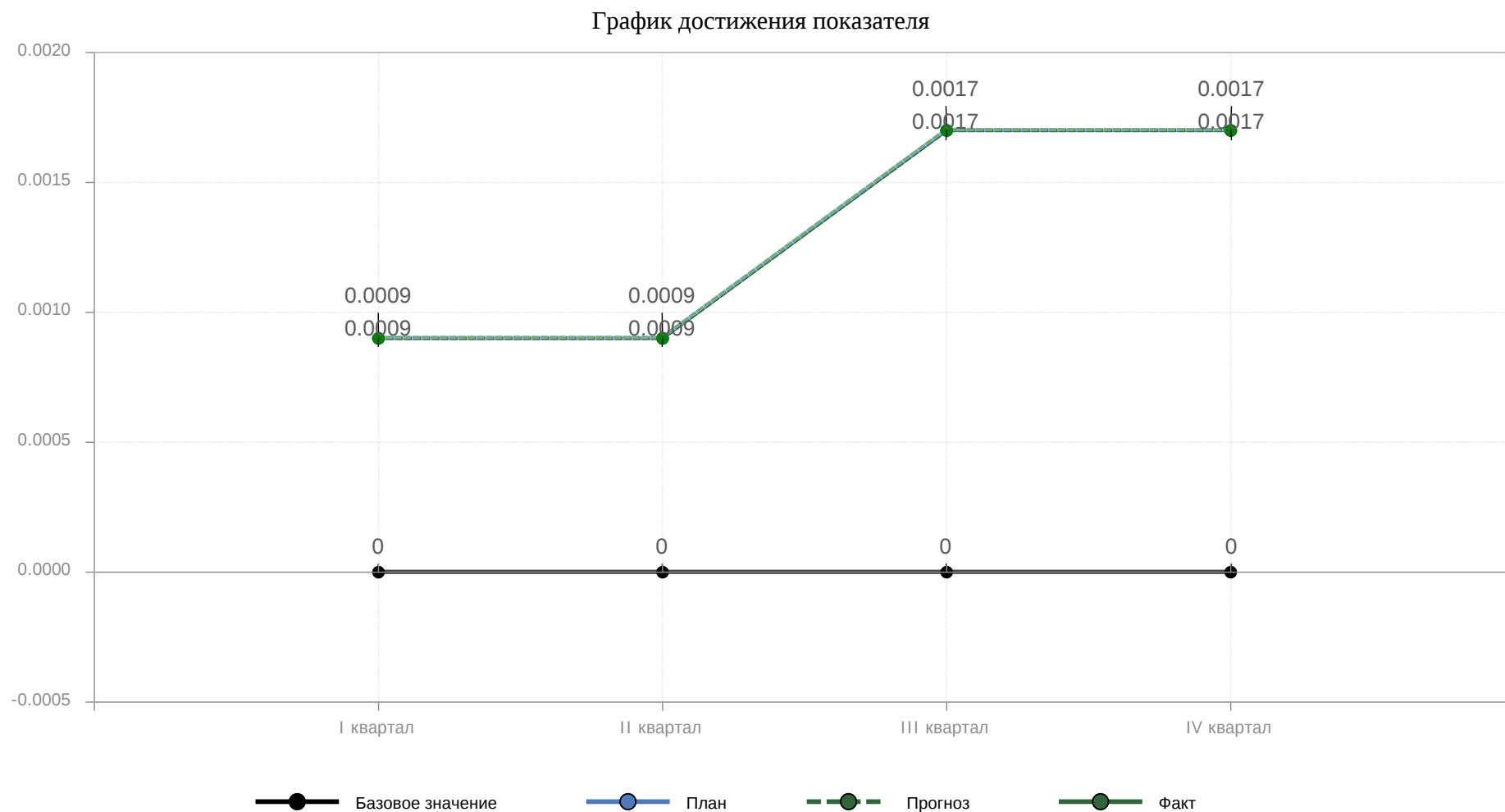
Рис. 3. Объем экспорта телекоммуникационных, компьютерных и информационных услуг
