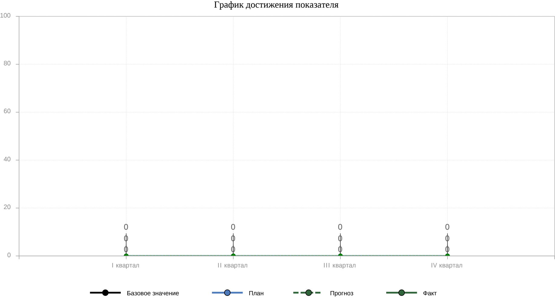
Рис. 13. Объем экспорта услуг частным лицам и услуг в сфере культуры и отдыха
